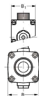
DEVSC25 DEVSC32 DEVSC40结构示意图
