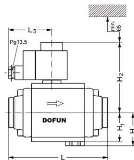
DEVSC25 DEVSC32 DEVSC40结构示意图
